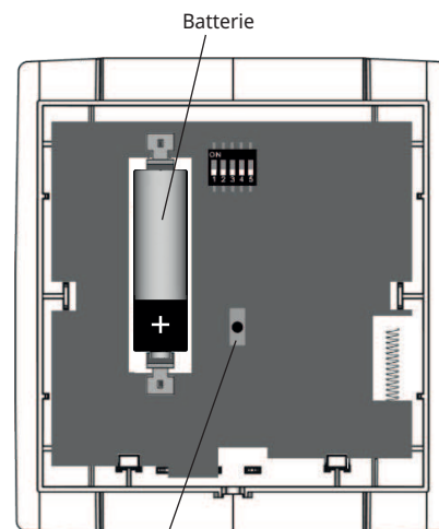
„Lernen“-Taste: um den Fühler mit Gateway zu verbinden/zu paaren
