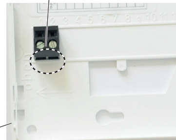
Pohjalevy; verkkosovittinjohtojen liittämä
