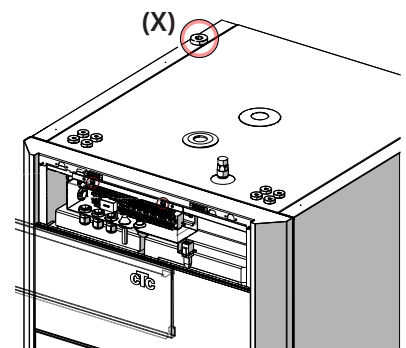
Positionnement du câble d'alimentation.
