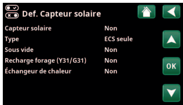
Menu : «Avancé/Définir/Capteur solaire».
