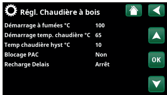
Menu : «Avancé/Réglages/Chaudière à bois».
