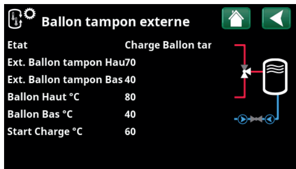
Menu «État opération/Ballon Tampon, externe».
