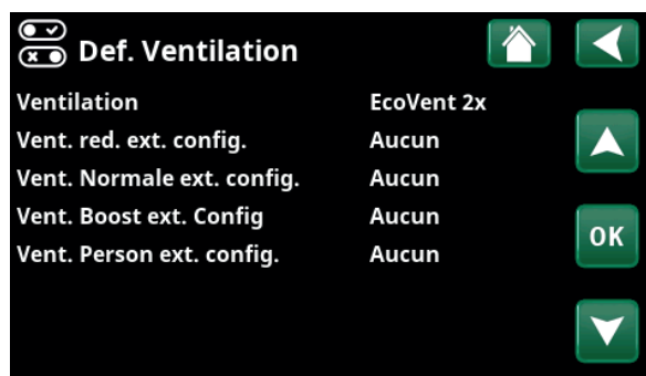
Menu : «Avancé/Définir/Ventilation».
