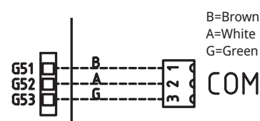
Gros plan du schéma de câblage.
