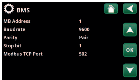
Menu : «Avancé/Réglages/Communication/BMS»
