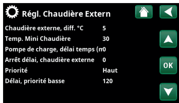
Menu : «Avancé/Réglages/Chaudière externe».
